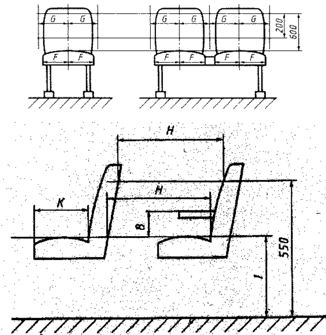
Рисунок 1.16.1. Размеры и расположение сидений
